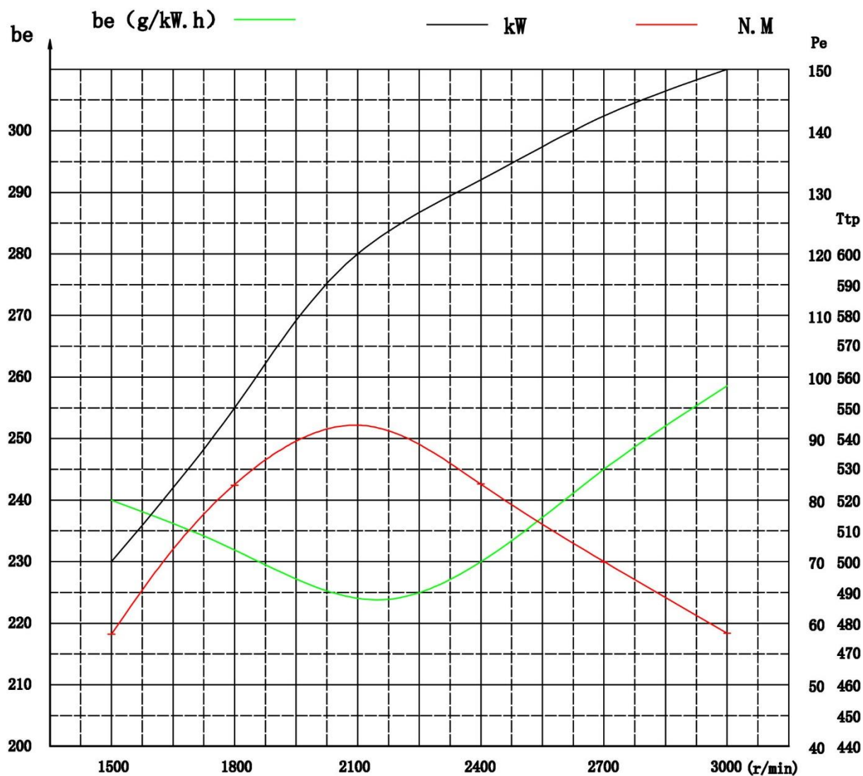
6BD-ZL特性曲线图
