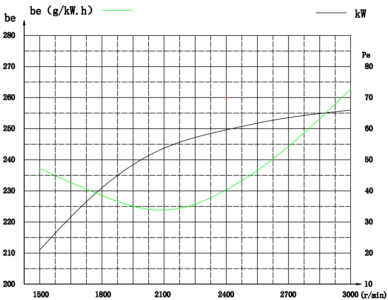
4BD-G 3000转特性曲线图
