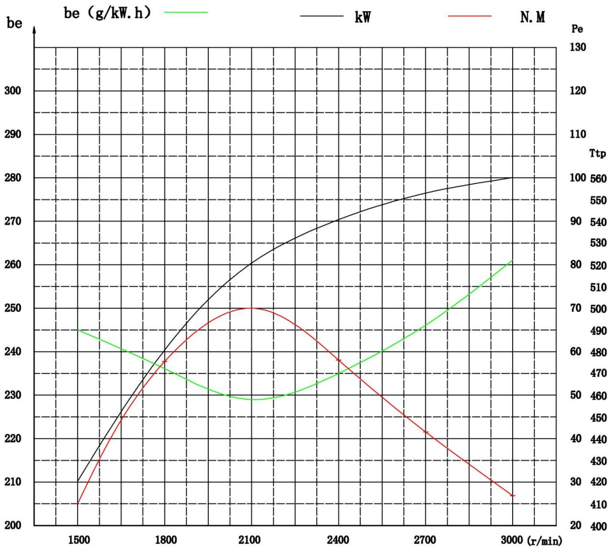
4BD1-ZLG特性曲线图
