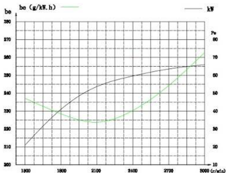
4BD-G 3000转特性曲线图
